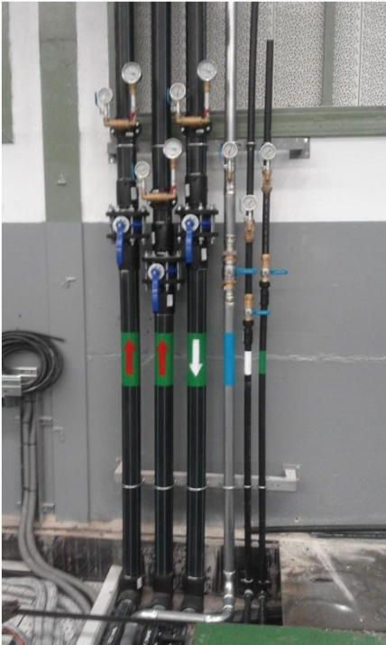
INSTALACION CIRCUITOS AGUA EN PROCESO COMPONENTES VILANOVA
